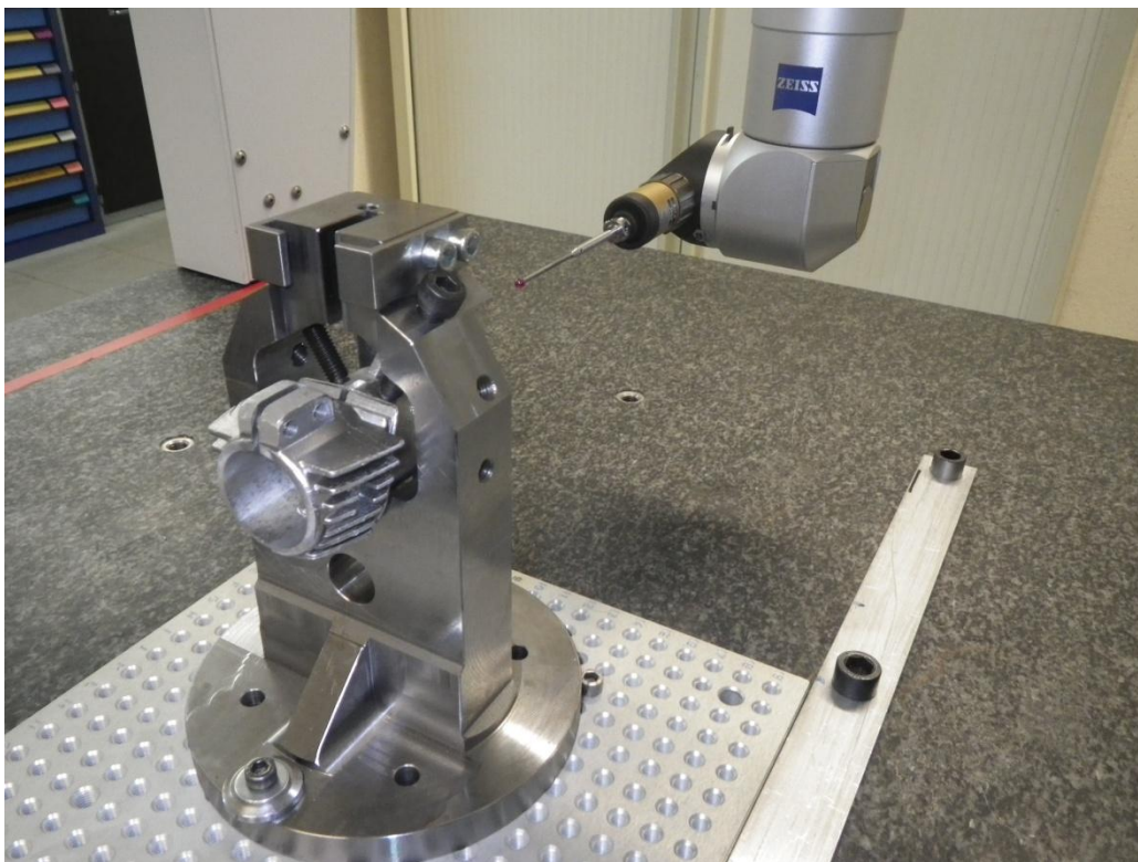
Outillage de fabrication et contrôle de composant de fonderie usiné
